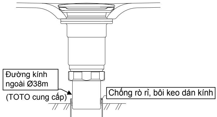
Sơ đồ lắp đặt
